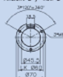
Ansicht B / view B
